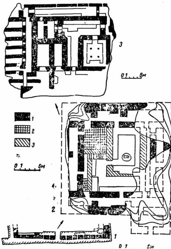
Рис. 1. Планы замков: 1—Кучуктепа (ю.-в. фасад), 2—Балалыктепа (по Л. И. Альбауму), 3—Джумалактепа (по В. А. Нильсену). Условные обозначения: 1—первый строительный период, 2—второй строительный период, 3—третий строительный период.
