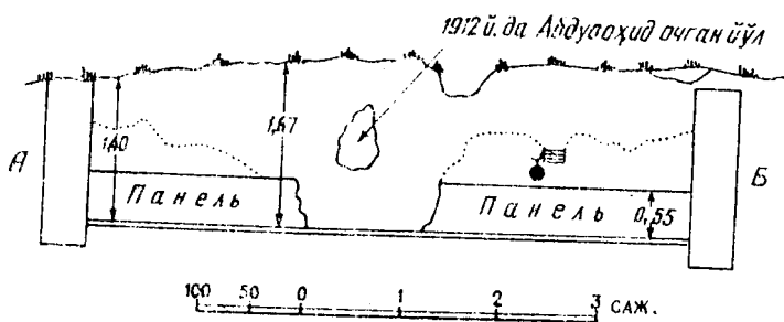
Ганч панелли зал АБ кесмасида.
