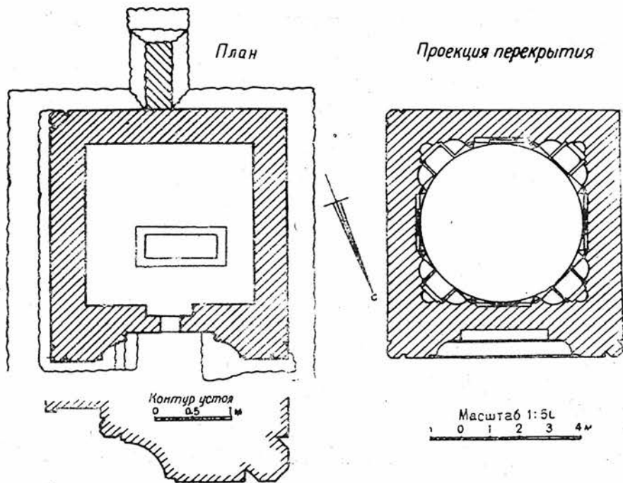
Рис. 3. План мавзолея и проекции перекрытия.
