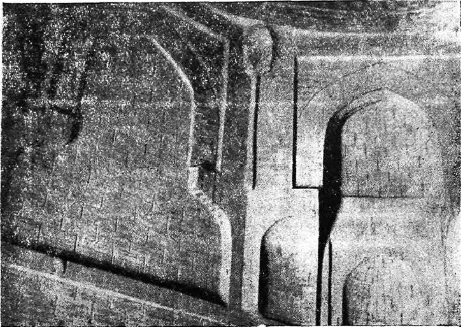
Рис. 2. Трехлопастные паруса подкупольной конструкции.
