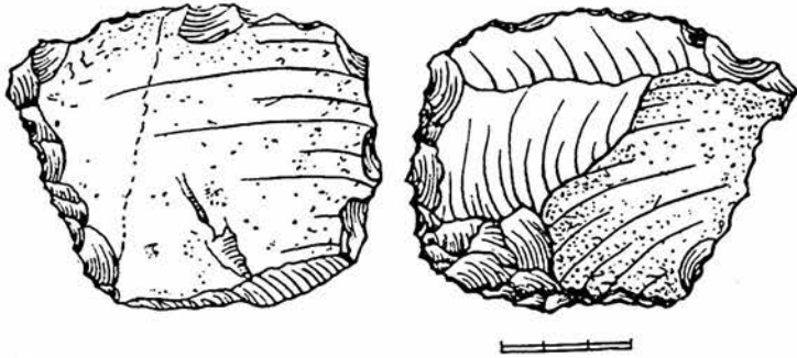
Рис. 1. Скребловидное орудие.
