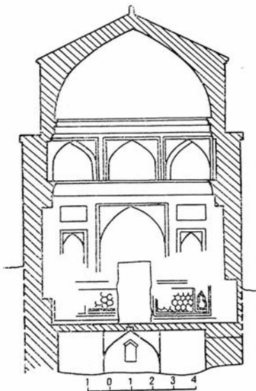
Рис. 2. Разрез мавзолея и склепа по линии север—юг.
