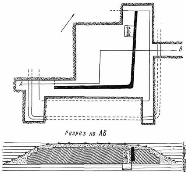
Рис. 1. Джандавлаттепа. Общий план и разрез по линии АВ.
