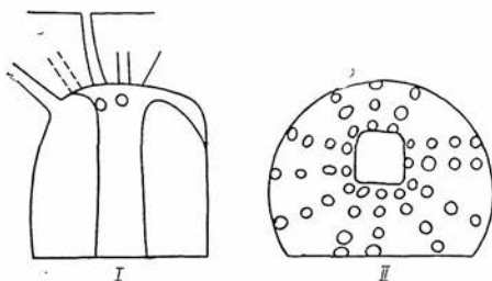
Рис. 1. Гончарная печь с Бауртена. I — разрез, II — план свода топки.
