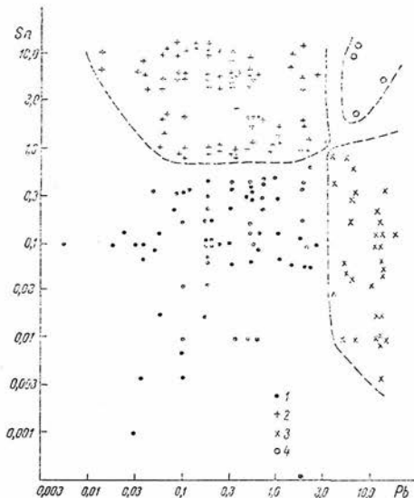
Рис. 2. Корреляционный график взаимозависимости концентраций олова и свинца в сапаллитепянской меди (по данным 194 анализов).
