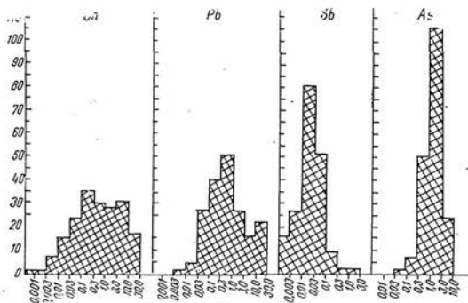
Рис. 1. Гистограммы распределения концентраций олова, свинца, сурьмы и мышьяка в сапалитенинской меди (по данным 194 анализов).
