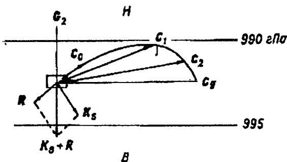
44-расм. Атмосферанинг чегаравий қатламида шамол тезлиги ва йўналишининг баландлик бўйича тақсимоги (шимолий яримшар).
