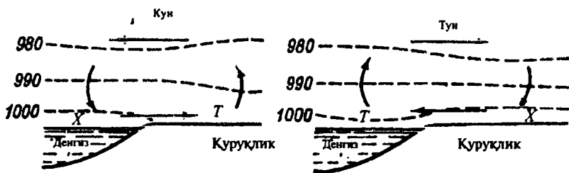
46-расм. Бризлар схемаси.
