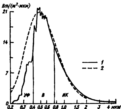
14-расм. Атмосферага киргунга қадар қуёш радиацияси спектридаги (1) ва 6000 К ҳароратли мутлақ қора жисм спектридаги (2) энергия тақсимооти. Спектр соҳалари: УВ – ультрабинафша, К – кўринувчан, ИҚ – инфрақизил.
