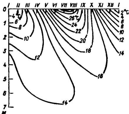
21-расм. Тупроқ ҳарорати йиллик ўзгаришининг изофлеталари.
