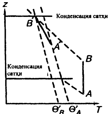
11-расм. Потенциал нотурғунлик
