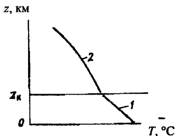
8-расм. Нам ҳавонинг ҳолат эгри чизиғи. 1 - қуруқ адиабата, 2 - нам адиабата.
