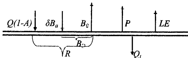
20-расм. Ер сирти балансининг сутканинг кундузги вақтидаги гашкил этувчилари.
