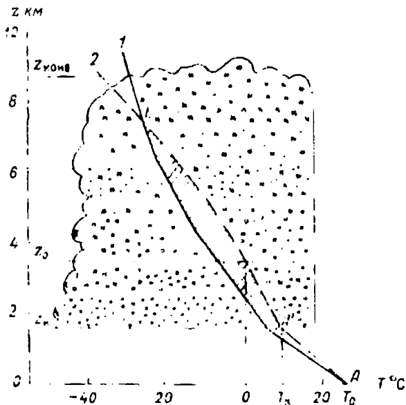
32-расм. Тўп-тўп ёмғирли булут схемаси. 1 – стратификация эгри чизиғи, 2 – ҳолат эгри чизиғи.
