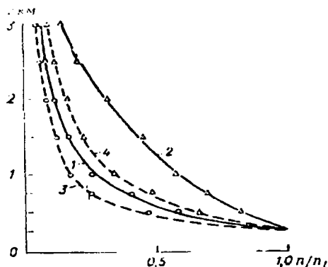
30-расм. Конденсация ядроларининг вертикал тақсимоги (1960-1964 йй. учун ўртача).
