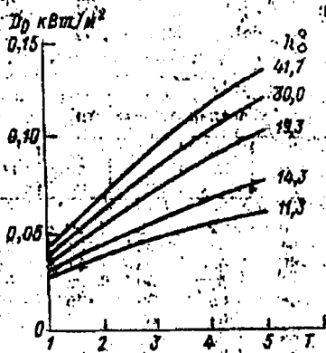
17-расм. Булутсиз осмонда сочилган радиация интенсивлигининг куёшнинг турли баландликларидаги h_{\odot} хиралик омили T га боғлиқлиги.
