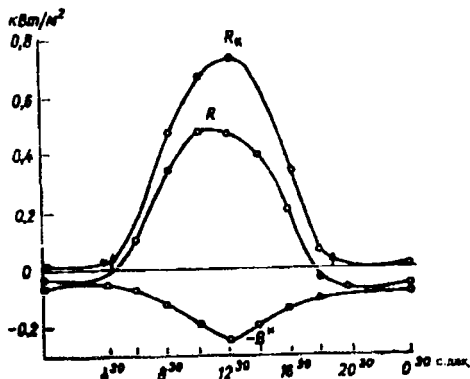
18-расм. Радиация баланси R , унинг узун тўлқинли R_k ва қисқа тўлқинли R_n ташкил этувчиларининг суткалик ўзгаришлари (Қозоғистон жануби, июл 1952 й.). Стрелкалар – Куёшнинг чиқиш ва ботиш вақтлари.
