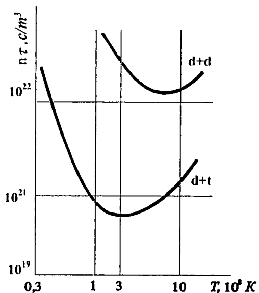
5.15-rasm. Deyteriy-tritii, deyteriy-deyteriy reaksiyalari uchun plazmani ushlab turuvchi parametrlarning temperaturaga bog'liqligi.
