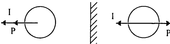
1.11-rasm. Ko'zgu aksiga ( P -ko'zguna) nisbatan impuls ( P ) ning va harakat miqdori momenti ( I ) ning o'zgarishi.
