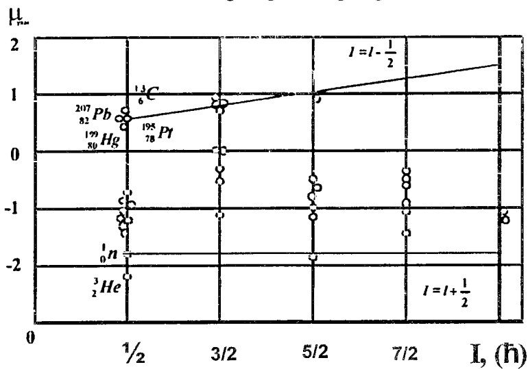
1.6-rasm. Toq neytronli yadrolar magnet momentlarining spinlari orasidagi bog‘lanish grafigi.
