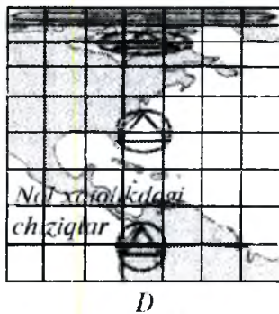
2.6-rasm. Silindrik proyeksiyalarda tuzilgan kartalardagi xatoliklar ellipsi: A – teng burchakli; B – teng maydonli (yoki ekvivalent); D – ixtoriy (teng oralig'li). Xatoliklar ko'rgazmali bo'lishi uchun aylana ichiga teng tomonli uchburchak chizilgan.
