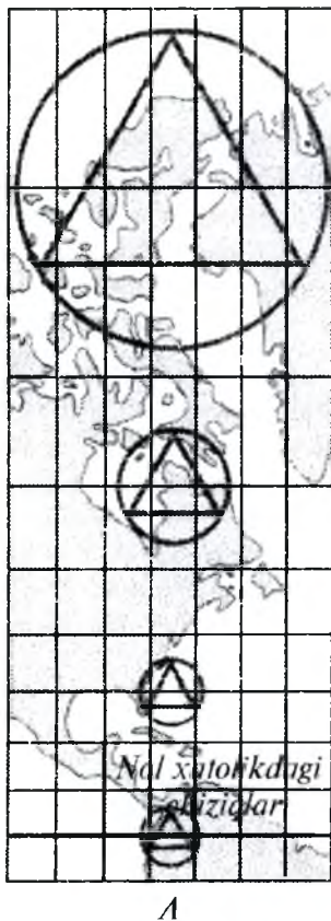
2.6-rasm. Silindrik proyeksiyalarda tuzilgan kartalardagi xatoliklar ellipsi: A – teng burchakli; B – teng maydonli (yoki ekvivalent); D – ixtoriy (teng oralig'li). Xatoliklar ko'rgazmali bo'lishi uchun aylana ichiga teng tomonli uchburchak chizilgan.
