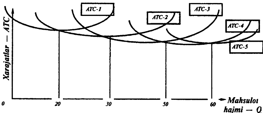
61-chizma. Turli yiriklikdagi korxonalariga qo'llaniladigan qisqa muddatli harajatlar egri chizig'i.
