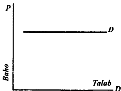
68-chizma. Sof raqobat bozorida talab hajmi.
