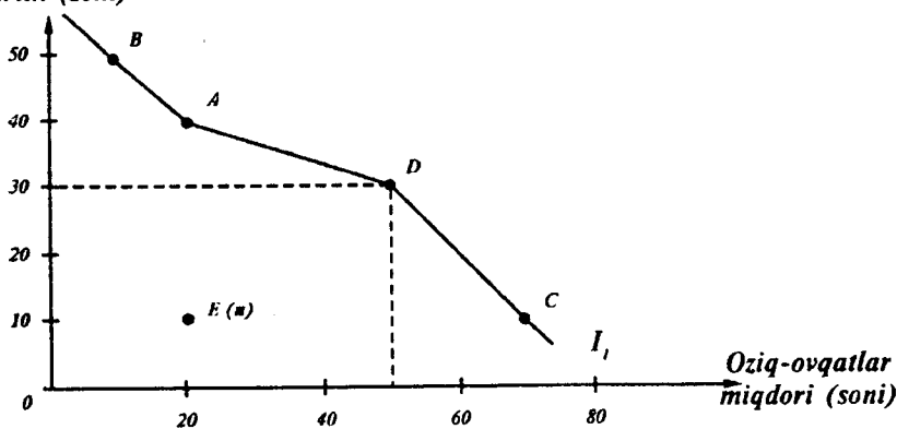
24-chizma. Befarqlik egri chizig'i.
