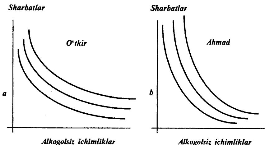
28-chizma. Tovar yoqtirishdagi individual farqlar.
