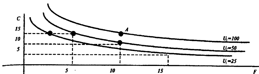
33-chizma. Befarqlik egri chiziqlari.
