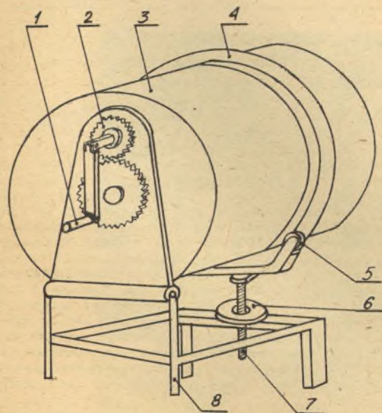
БЕТОН ҚОРУВЧИ (1-хил) 1-айлантиргич 5-галтакча 2-тишли гилдирак 6-гилдиракча 3-бўчка 7-мурувват 4-айланиш сирти 8-таянч
