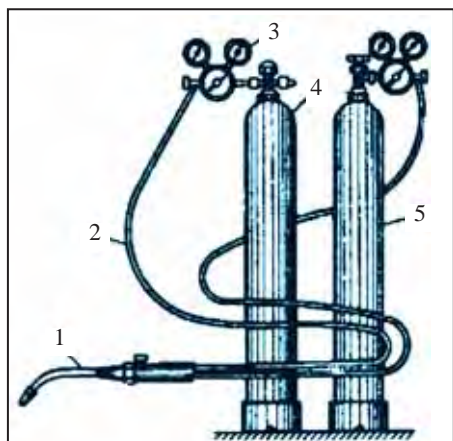
26-su'wret. Gaz benen kepslerew ushi'n u'skeneler: 1-gorelka; 2-shlanglar; 3-reduktor; 4-kislorodli' ballon; 5-acetilenli ballon.
