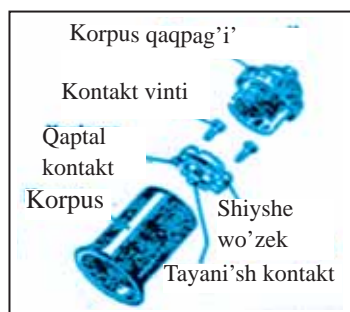
77-su'wret. Aspa patronni'n' du'zilisi.
