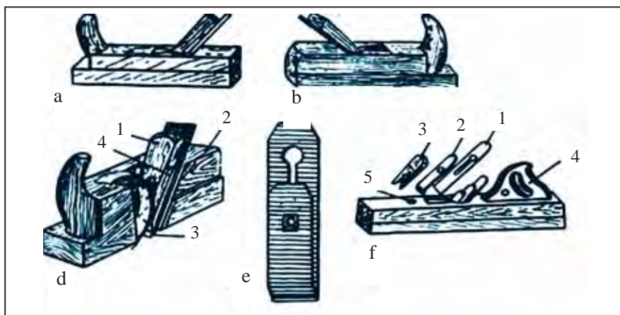
50-su'wret. Su'rginin' tu'rleri: a) sherxebel; b) taxta su'rgi; d) mushsu'rgi: 1-si'na; 2-denesi; 3-ju'zi; 4-temir si'na; e) temir si'nali' ju'z; f) japs su'rgi: 1-ju'zi; 2-temir si'na; 3-si'na; 4-tutqa; 5-balg'alaw tu'yini.
