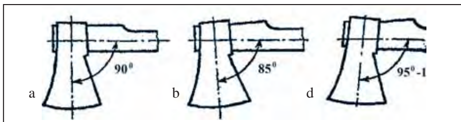
56-su'wret. Balta ju'zinin' tutqasi'na sali'sti'rg'anda jaylasi'wi': a) tuwri' mu'yesh asti'nda (woti'n jari'w ushi'n); b) su'yir mu'yesh asti'nda (shaqalardi' shabi'w ushi'n); d) dog'al mu'yesh asti'nda (terekti biraz shawi'p qoyi'w ushi'n).
