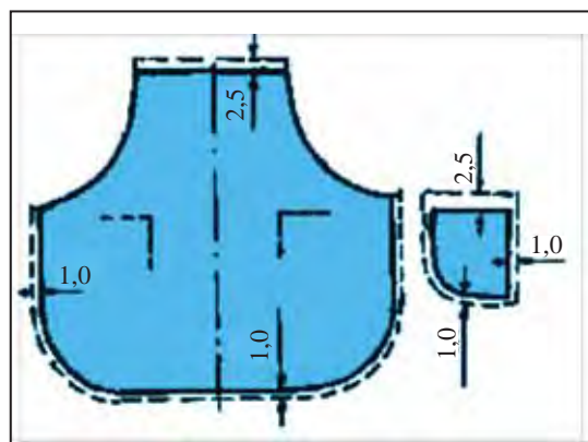
44-su'wret. Fartuk detallari'.
