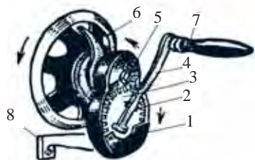
28-su'wret. Qolda ju'rgiziw bo'limi.
