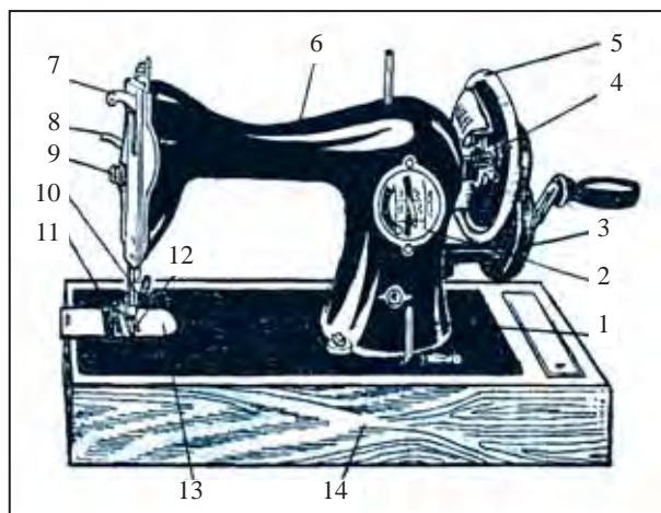
27-su'wret. Qolda ju'rgizetug'i'n tigiw mashinasi'ni'n' tiykarg'i' bo'limleri.
