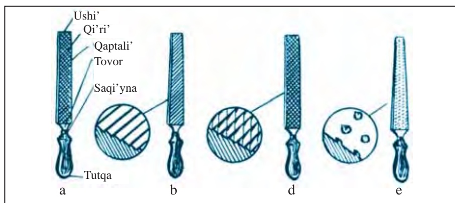
59-su'wret. Yegewlər: a) du'zilisi; b) bir qi'rli'; d) yeki qi'rli'; e) noqat qi'rli'.
