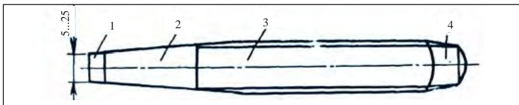
10-su'wret. Tokarli'q zubilosi'. 1–ju'zi. 2–jumi's bo'limi. 3–worta bo'limi. 4–basi'.
