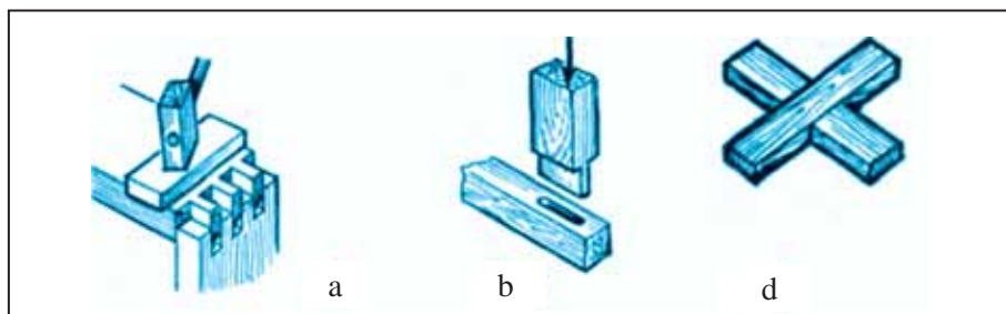
62-su'wret. Ti'rnaqli' birikpelerdi ji'ynaw: a) tuwri' ti'rnaq; b) «T» ta'rizli ti'rnaq; d) ashi'q ti'rnaq.
