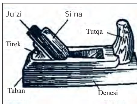
51-su'wret. Su'rginin' du'zilisi.
