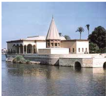
Ahmed Ferganiy tärepinen qurılğan Nil dáryasında suw qáddin ólsheytuǵın qurılma. Sırtqı hám ishki kórinisi. IX ásir
