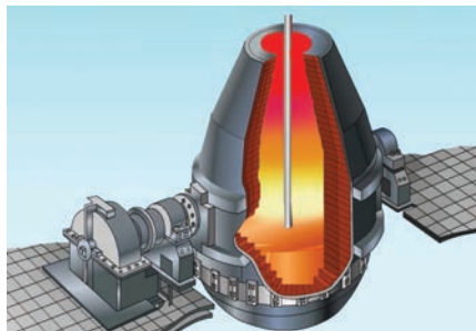
Расми. 19. Қонвертори оксиген.
