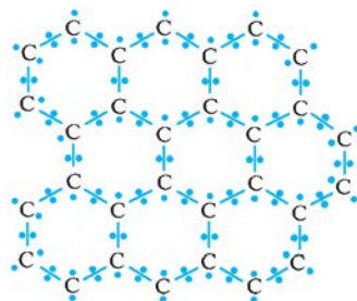
Расми 9. Сохти электрони графит.
