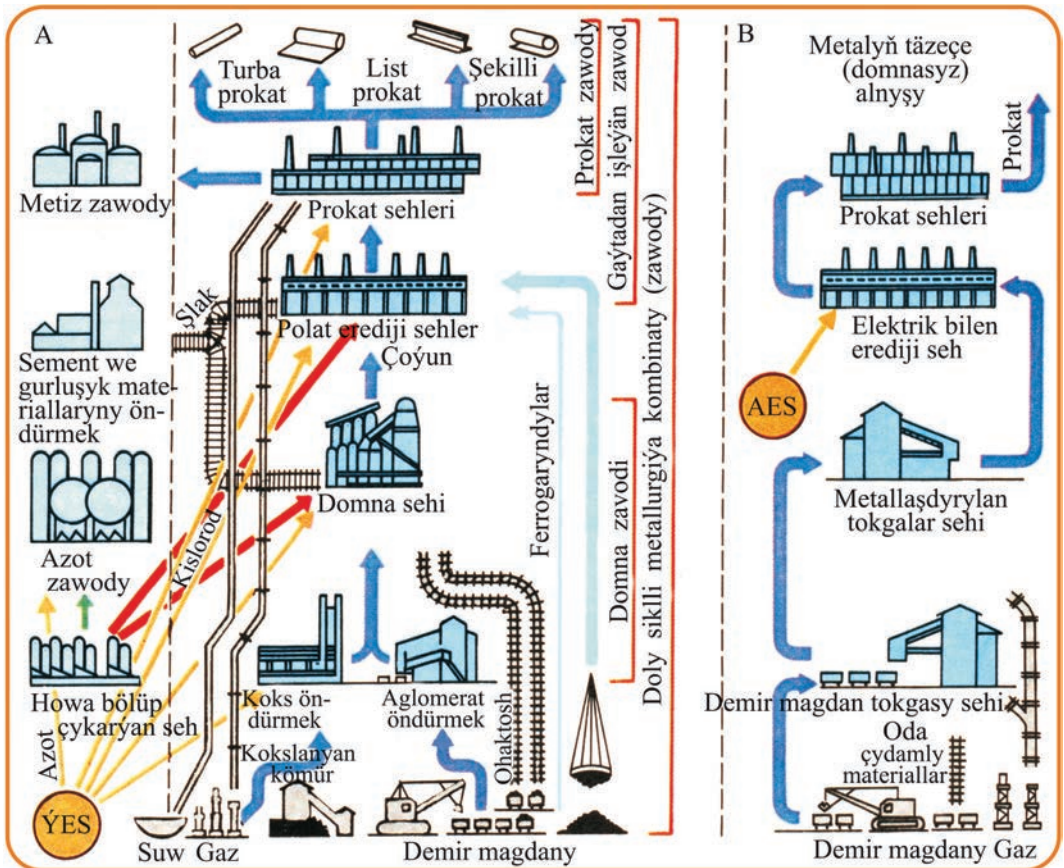
35-nji surat. Metallurgiýa kombinatyndaky sehleriň shemasy.
