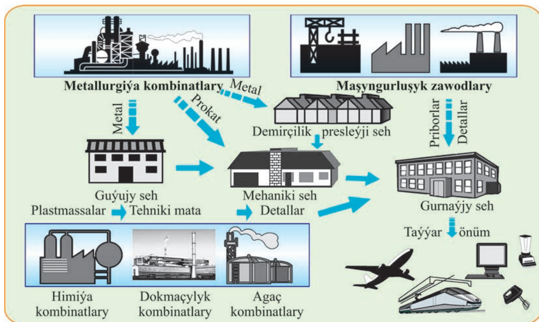
41-nji surat. Maşyngurluşyk zawodynyň düzümi.
