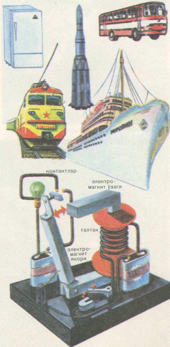
Электроманнит реле. Унинг ғалтаги орқали ток ўтказилса, якорь ўзакка тортилиб, контактлар бирикади ва лампочка ёнади.
