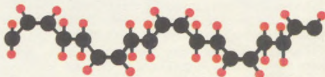
каучук молекуласи
