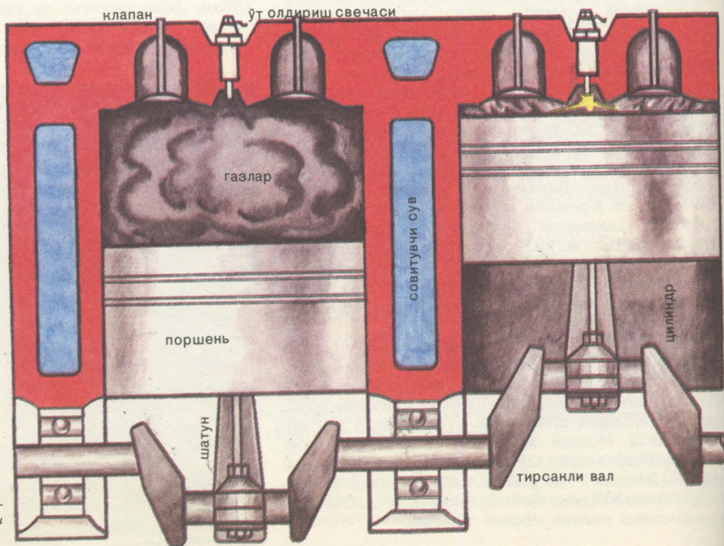
Суратда ички ёнув двигателининг қандай ишлаши тасвирланган.
