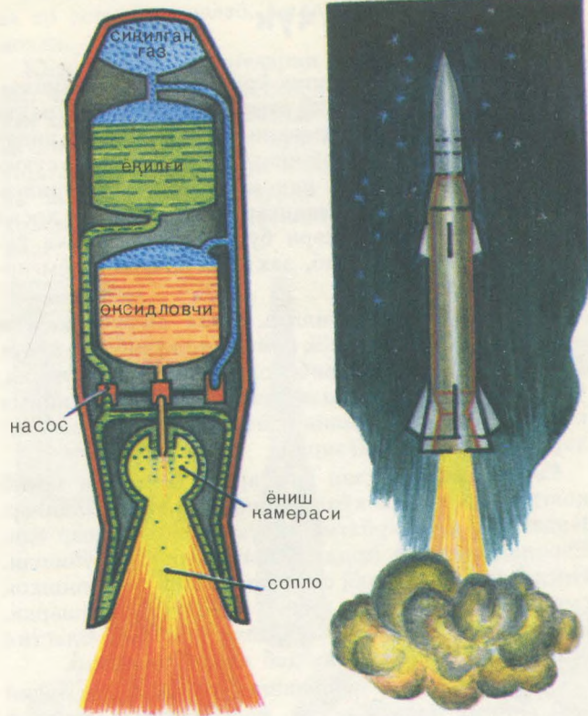
суюқ ёқилғида ишлайдиган реактив двигателъ ўнгда: метеорологик ракета
