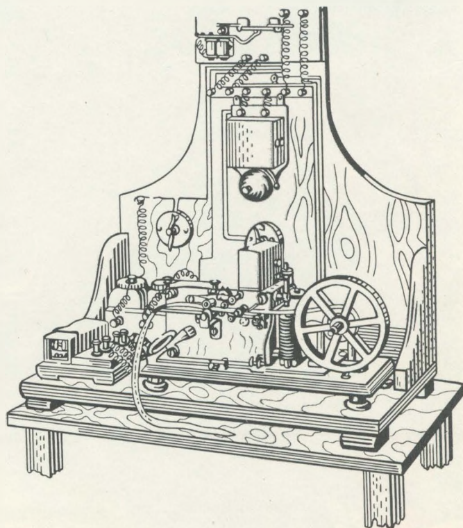
А. С. Поповнинг радиоприёмниги.
