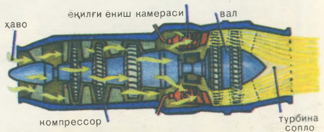
турбореактив двигателъ юқорида: товуш тўлқинидан тез учадиган самолёт
